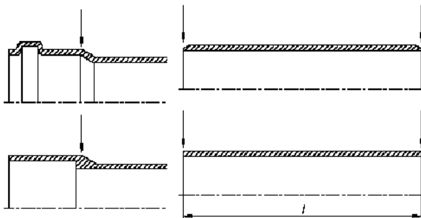
Fig.1.1-Standard di misurazione della lunghezza di tubi in PVC rigido
